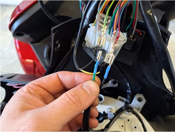
Irrota jarruvivun mikrokytkimen liittimet johtosarjasta.
